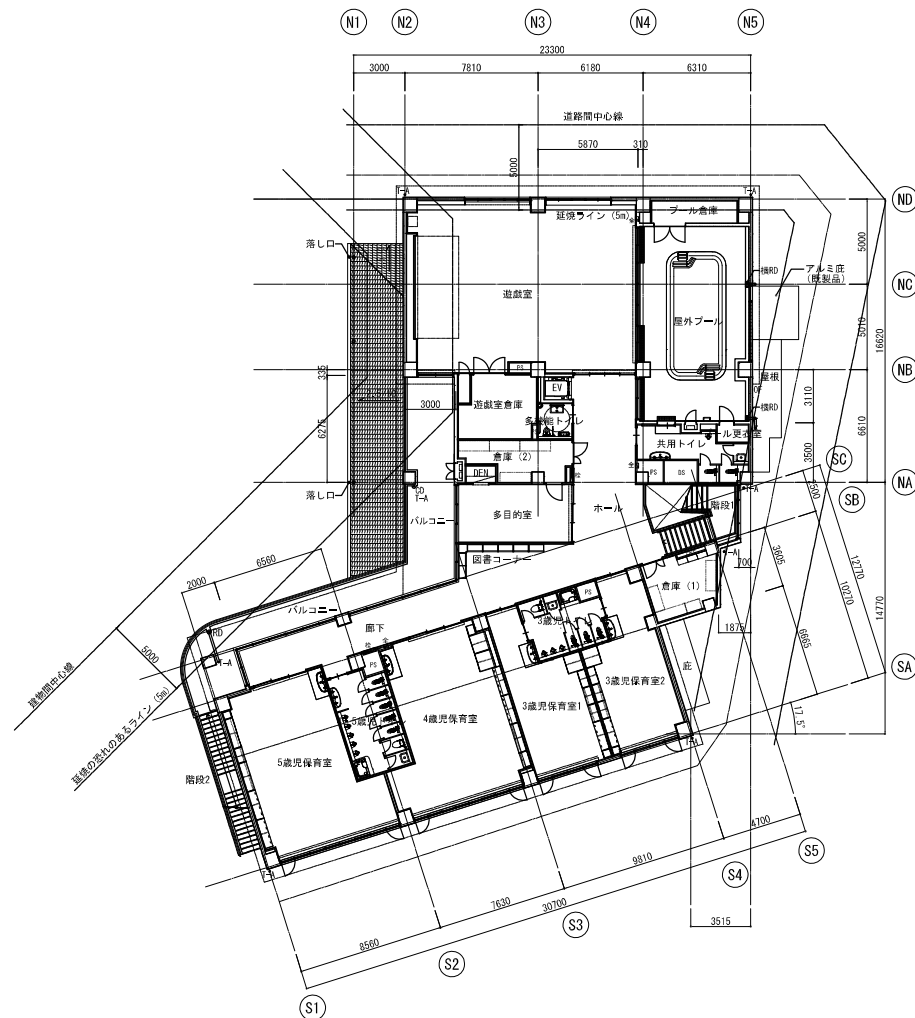
2階平面図
