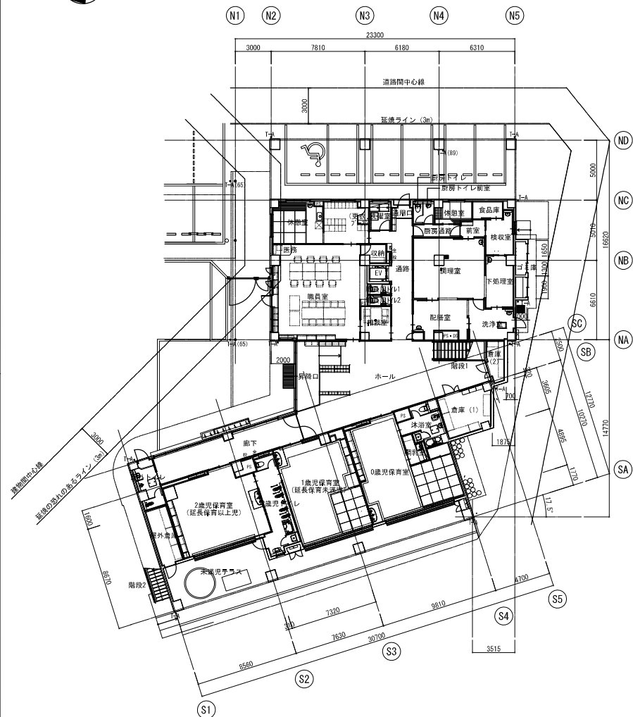
1階平面図
