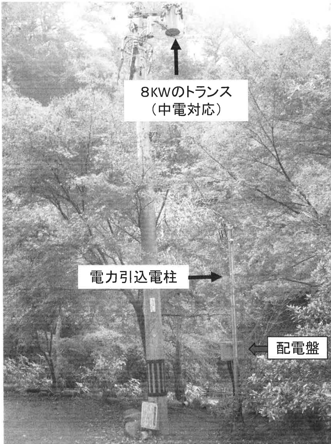
配電盤設置図
